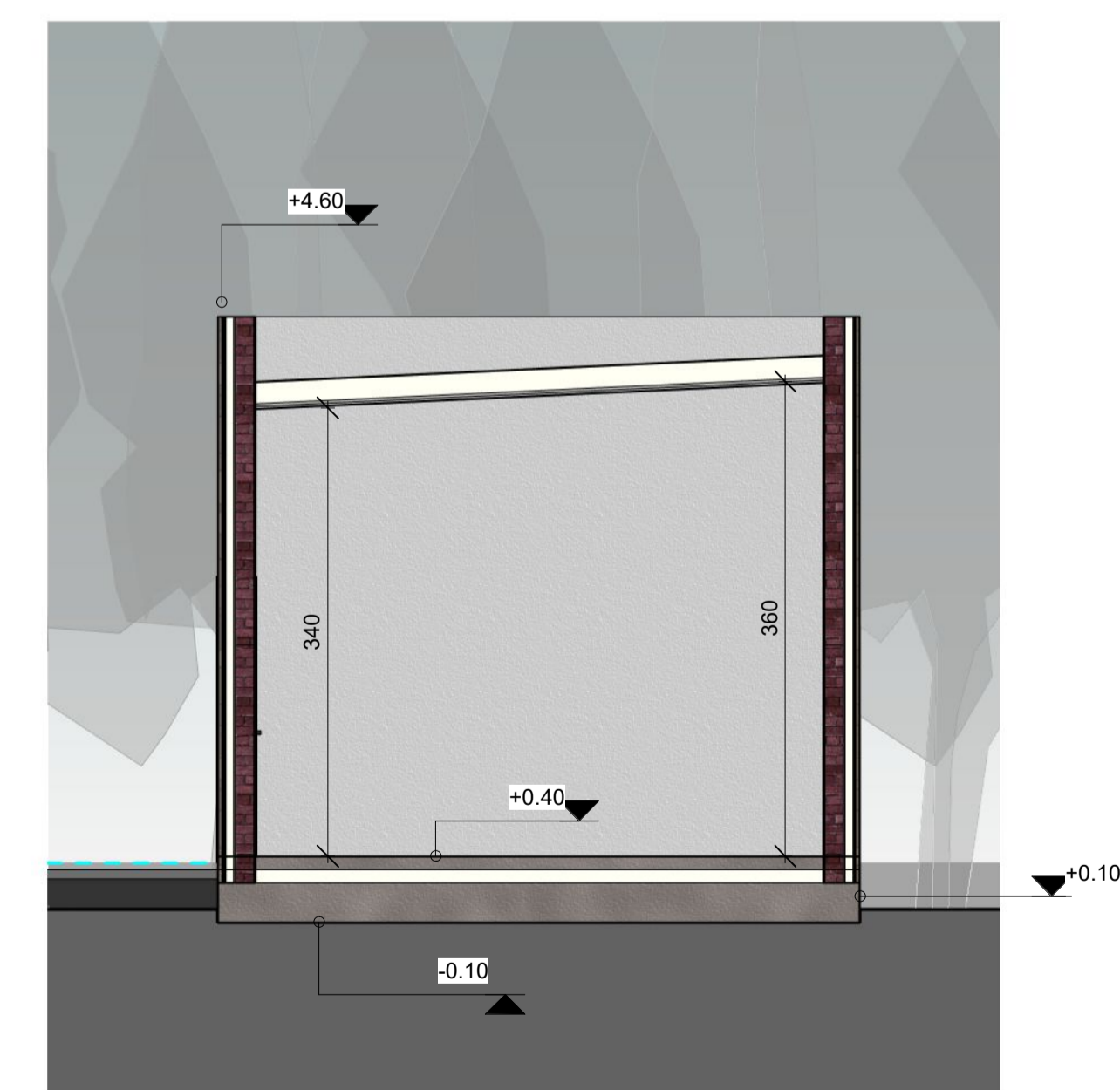
Locale Impianti - Sezione tipica
