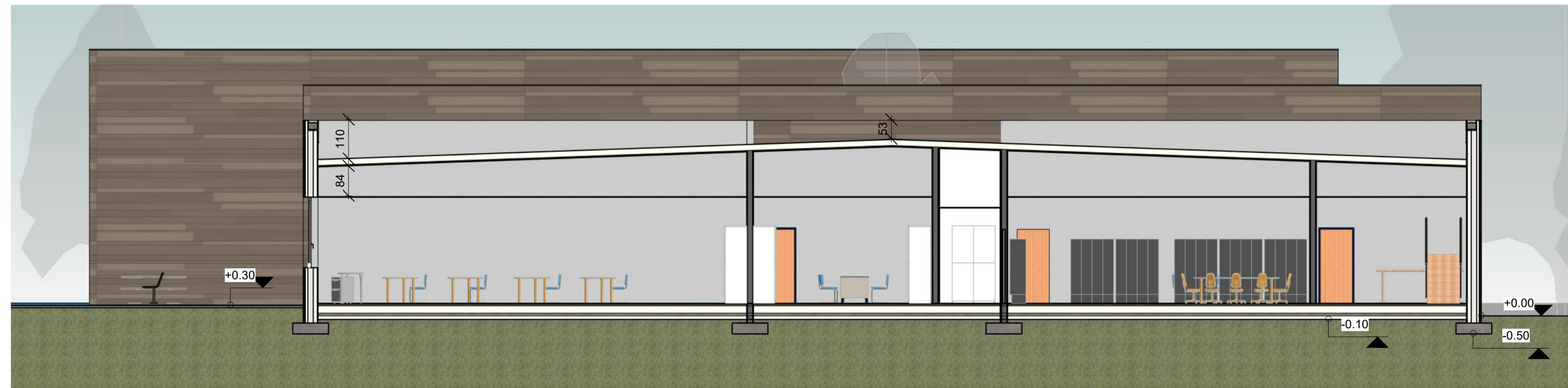
SEZIONE AA
